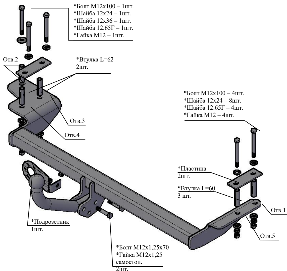
Рис.1 Тягово-сцепное устройство 9410
